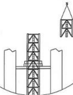
步驟十一:爬升塔節及標準塔節拆除
